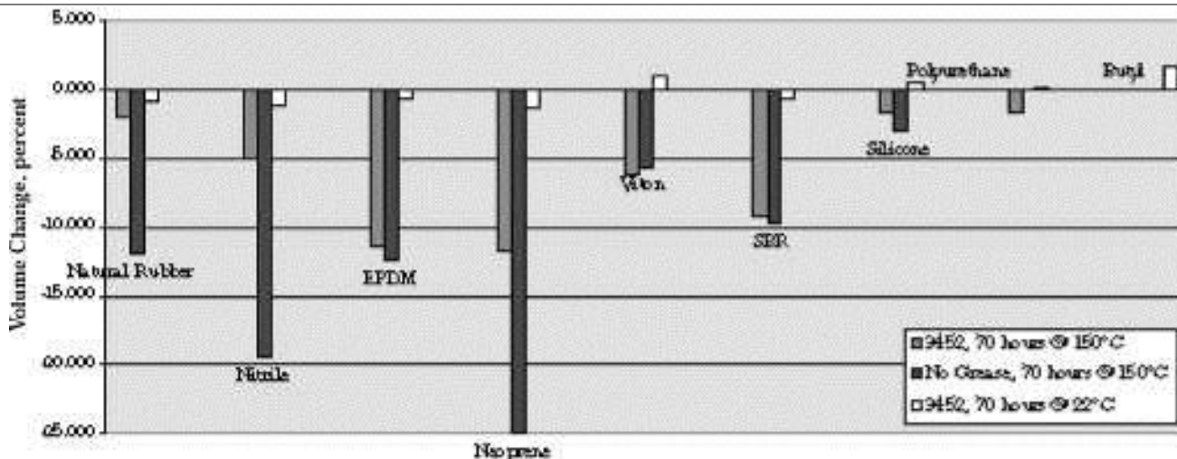
Рисунок 1: Изменение объема различных резин (в %) в устойчивой к химикатам смазке для вентилях MOLYKOTE 3452
